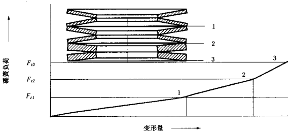
图 C.6 不同厚度的对合组合碟簧
