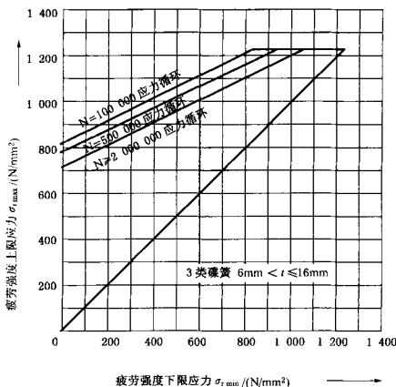
图 C.11 6 mm < t ≤ 16 mm 碟簧的疲劳强度曲线图
